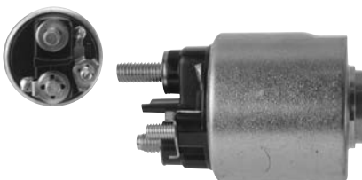
236975 Solenoid Replacing: 594414 Servicing: D6RA137, d6ra138, D6RA187, D6RA188, D6RA87 12 V, B+ M8, Kl. 50 M6, OD 54.00, OD/ cover 46.00, Total length 89.30, Height/ B+ 17.50, Width/ kl. 50 10.81, Coil bolt M8, Coil bolt 2 M8, No./ terminals 3
