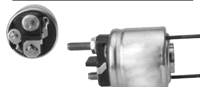
330689 Solenoid Replacing: 594724 Servicing: D6G5 12 V, B+ M8, Kl. 50 M6, OD 54.29, Total length 89.46, Height/ B+ 20.80, Width/ kl. 50 7.37, Coil bolt M8, Coil bolt 2 9.32, No./ terminals 3
