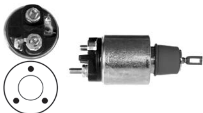
232186 Solenoid
