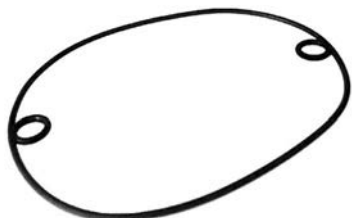
135580 Gasket Replacing: 2000290012 Servicing: 0001362321, 0001362331, 0001363128, 0001363130, 0001367036, 0001367038, 0001367046, 0001367051, 0001367054, 0001367057 Thickness 1.20, Material Rubber
