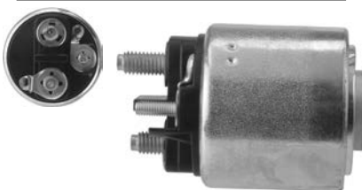
237686 Solenoid Servicing: D7E39, TS8E6 12 V, B+ M8, Kl. 50 M5, OD 54.00, Total length 59.00, Height/ B+ 14.50, Width/ kl. 50 10.00, No./ terminals 3
